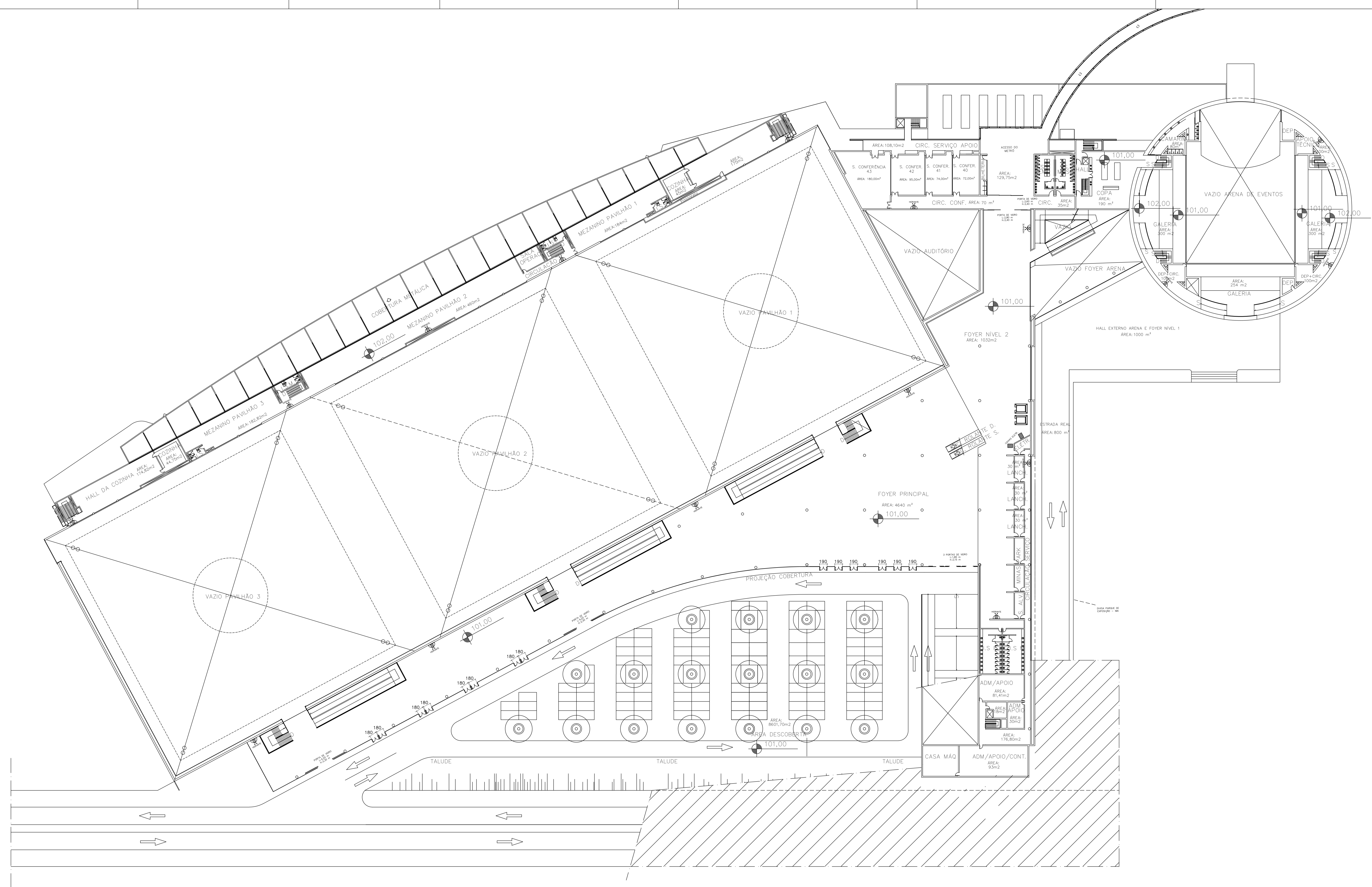
PLANTA 2º PAVTO
